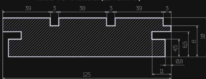
Панель «FD» 3 полосная (125 x 2750 мм)
