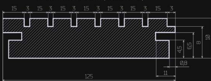
Панель «FD» 7 полосная (125 x 2750 мм)
