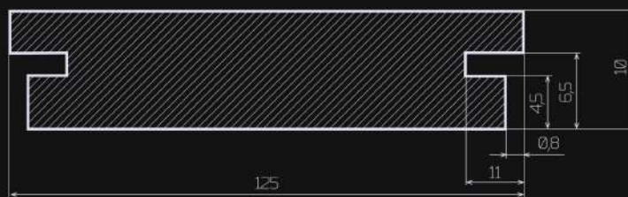
Панель «FD» 125 (125 x 2750 мм)
